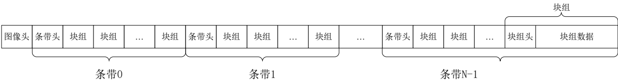
图4 增强层编码位流结构
