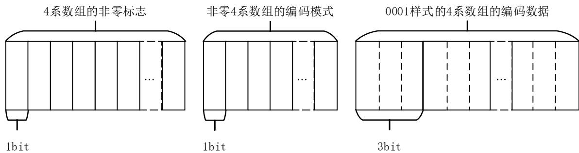
图9 块编码模式为 2 的 Z 编码数据结构示意图
