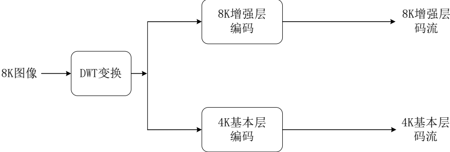
图2 8K 超高清视频浅压缩分层编码框架
